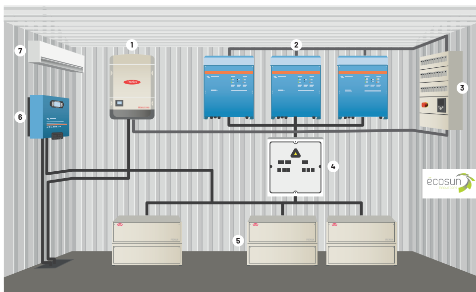
Exemple de la salle technique version container
