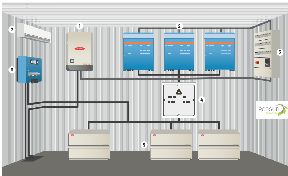
Schaltraum: Schematische Darstellung
